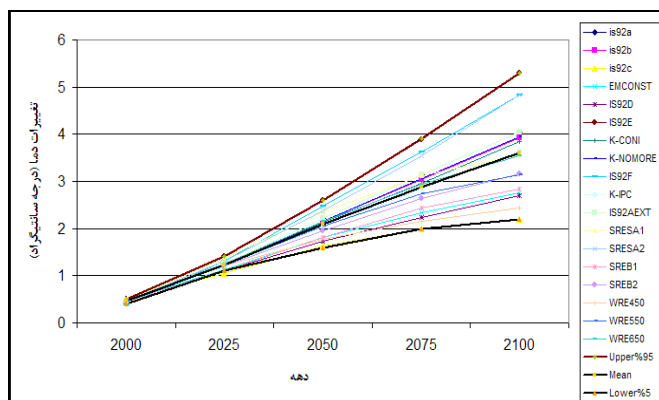
شکل ۱۱. برآورد تغییرات دمای دهه‌ای کشور توسط مدل M-S با استفاده از داده‌های مدل
