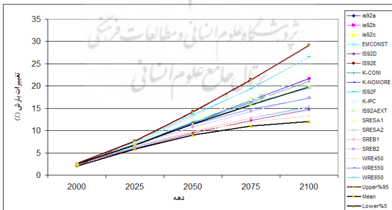
شکل ۵. بر آورد تغییرات دهه ای بارش کشور توسط مدل M-S با استفاده از داده‌های مدل
