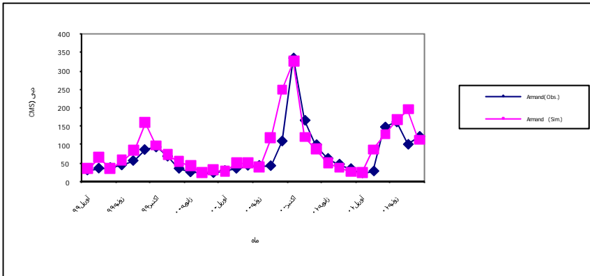
شکل ۶: مقایسه دبی ماهانه مشاهداتی و پیش بینی شده در ایستگاه ارمند
