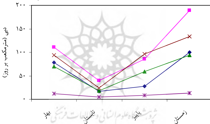
شکل ۲- مقادیر میانگین فصلی و ماهانه دبی رودخانه مارون در ایستگاه‌های مورد مطالعه (۱۳۶۸-۱۳۸۷)
