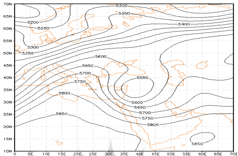
شکل ۲۱: نقشه ارتفاع تراز ۵۰۰ هکتوپاسکال (۹ فروردین ۱۳۸۸) ساعت ۰۰
