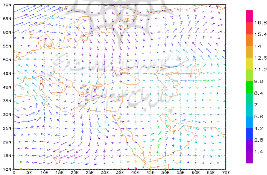
شکل ۲۶: وزش رطوبتی تراز ۸۵۰ هکتوپاسکال (۹ فروردین ۱۳۸۸) ساعت ۰۰ مأخذ: نگارندگان
