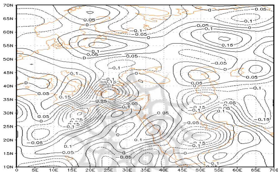
شکل ۹: اُمگا تراز ۸۵۰ هکتوپاسکال (۱۸ فروردین) ساعت ۱۲۰۰
