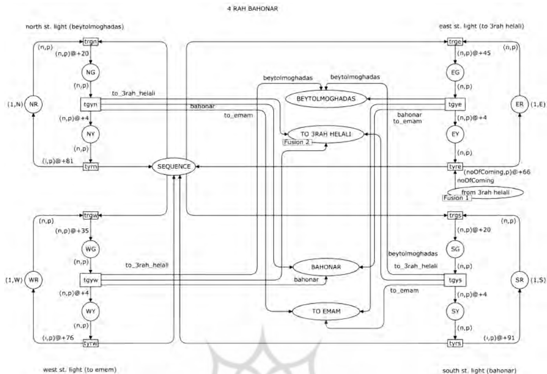
شکل شماره (۳): مدل شبکه پتری رنگین برای چهارراه باهنر
