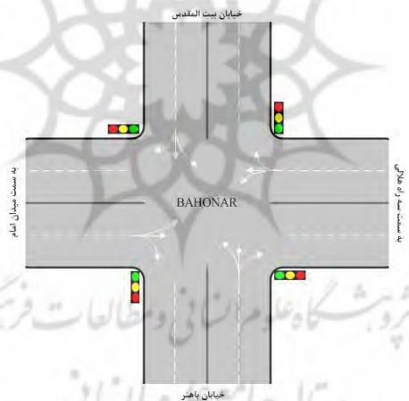
شکل شماره (۲): نمای کلی چهارراه باهنر
