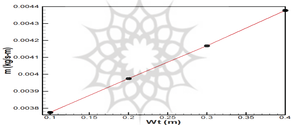
شکل ۸) تغییرات دبی جرمی عبوری از دریچه بالایی دیوار تورومب به ازای ضخامت‌های مختلف دیوار
