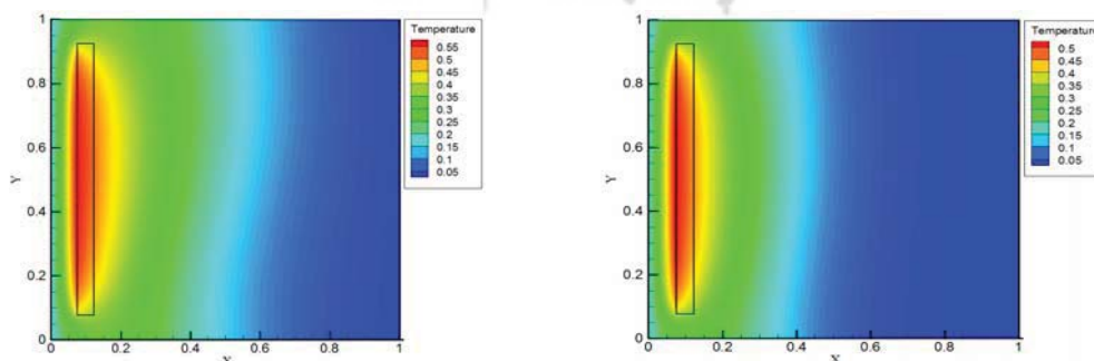
شکل ۱۱) توزیع دما و خطوط دما ثابت در زمان t=1000\text{s} (شکل ۱۲) توزیع دما و خطوط دما ثابت در زمان t=2000\text{s}
