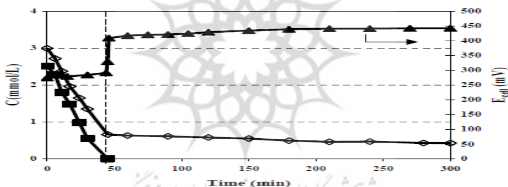
شکل ۴) فرایند شارژ در پیل الکتروشیمیایی ( کاتد: الکتروکود O_2 )،
