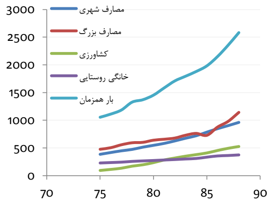
شکل ۲: حداکثر بار مصرفی (مگاوات) برق منطقه ای باختر از سال ۱۳۷۵ تا ۸۸
