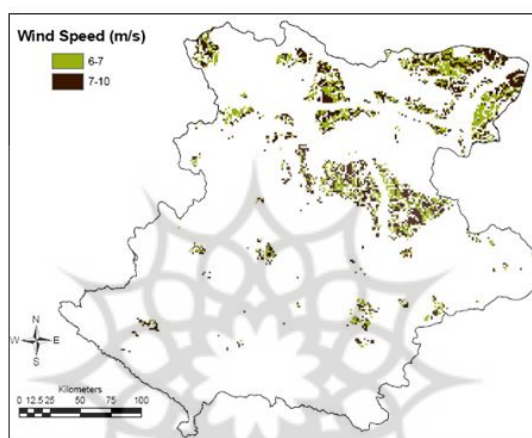
شکل ۹: نقشه پتانسیل سنجی باد برق منطقه ای باختر
