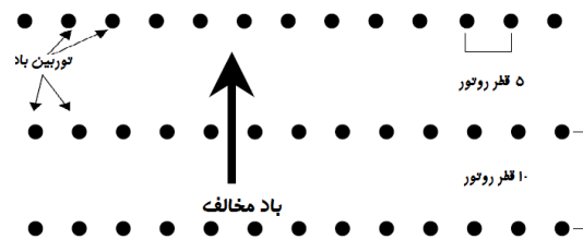
شکل شماره (۱۰) نحوه ی چیدمان توربین ها با روش Lissaman
