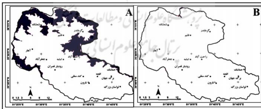
شکل 12 مقایسهٔ ارتفاع قلمرو مجاور یخچالی A: کوتاه‌تر 3000-3900 متر و B: زمان حال 4000-4220 متر
