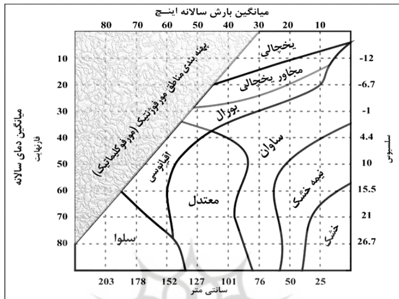
شکل 5 نمودار مناطق مورفوتنیک پلتیر
