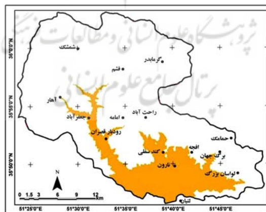
شکل 14 قلمرو پدیماناسیون در زمان حاضر، دامنه ارتفاعی 1565-2200 متر
