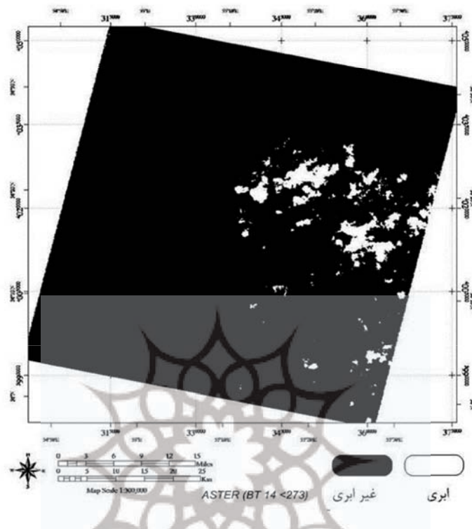
شکل ۵ نتیجه حاصل از آستانه‌گذاری تصویر BT ۱۴
