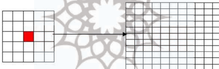
شکل ۳ نمایی شمانیگ از مقایسه یک پیکسل MODIS با ۱۱ در ۱۱ پیکسل ASTER
