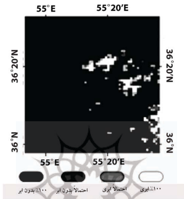
شکل ۱۵- درصد پوشش ابر به دست آمده از مدل
