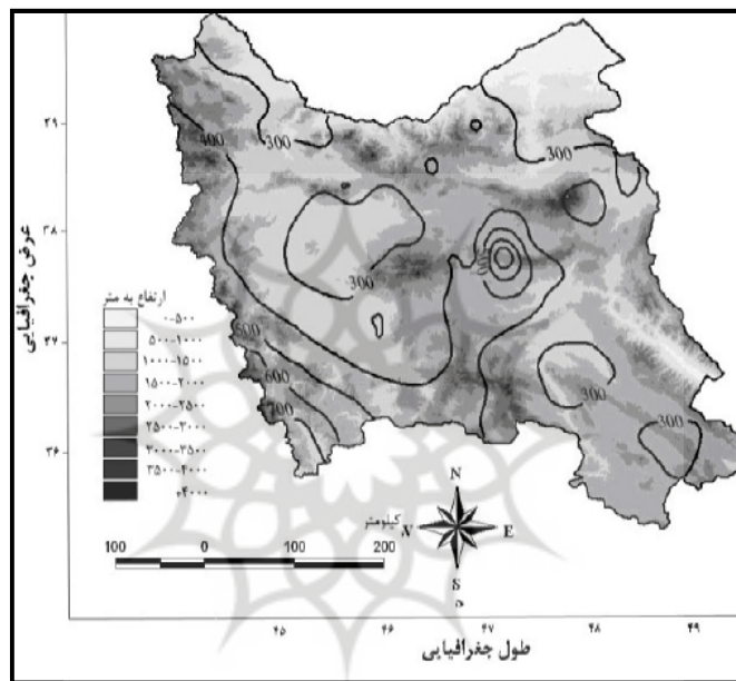
شکل ۵: توزیع مکانی بارش منطقه‌ی شمال غرب کشور تیرگی زمین‌ی نقشه گویای طیف ارتفاعی پهنه است.
