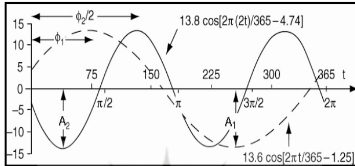
شکل ۳: همساز اول (خط چین) و دوم (خط ممتد) یک چرخه سالانه
