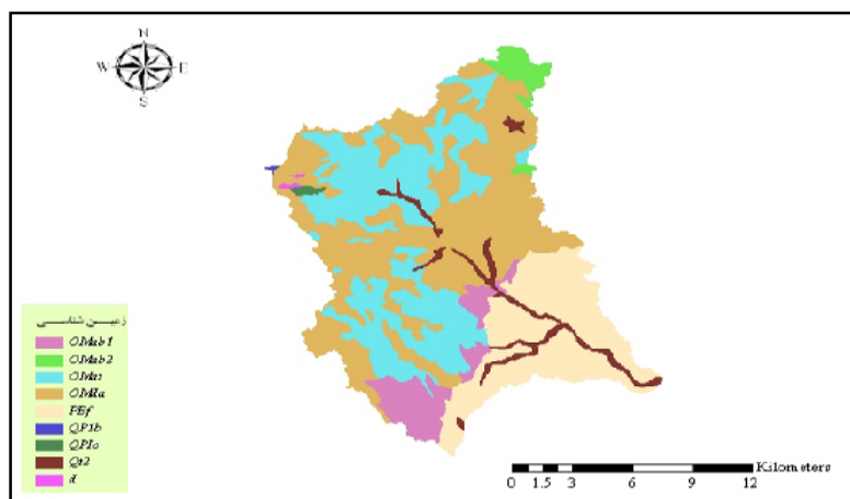
شکل ۶: نقشه زمین‌شناسی حوضه آبریز منصورآباد مأخذ: نگارندگان
