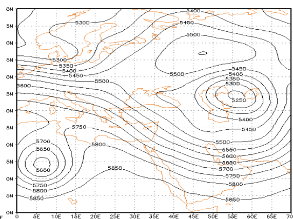
شکل ۱۷- نقشه ۵۰۰ هکتوپاسکال ۱۸ دی ۱۳۸۶ (ساعت ۰۰۰۰ UTC)
