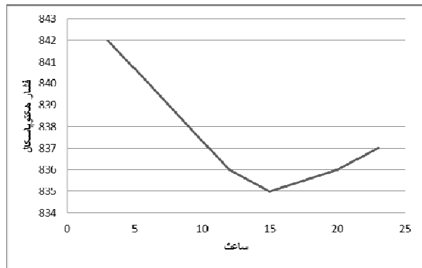
شکل ۱- تغییرات ساعتی فشار در روز ۱۷ دی ۱۳۸۶ ایستگاه سینه‌پتیک اصفهان
