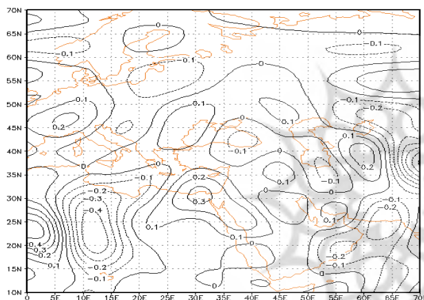
شکل ۲۰- نقشه امگای ۸۵۰ هکتوپاسکال ۱۸ دی ۱۳۸۶ (ساعت ۰۰۰۰ UTC)
