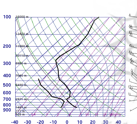
شکل ۸- نمودار ترمودینامیک روز ۱۷ دی ۱۳۸۶ (ایستگاه اصفهان)
