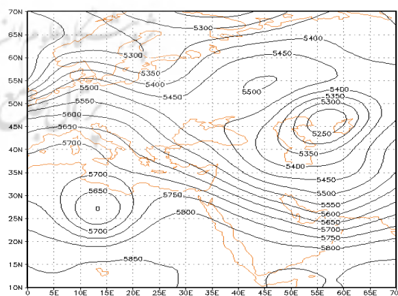
شکل ۲۳- نقشه ۵۰۰ هکتوپاسکال ۱۹ دی ۱۳۸۶ (ساعت ۰۰۰۰UTC)
