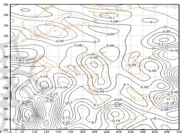
شکل ۱۹- نقشه امگای ۵۰۰ هکتوپاسکال ۱۸ دی ۱۳۸۶ (ساعت ۰۰۰۰ UTC)
