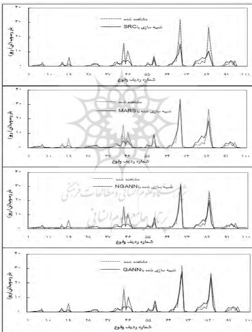
شکل ۵- مقایسه اختلاف خطای بین مقادیر مشاهده شده و مقادیر پیش‌بینی شده رسوب در روش‌های چهارگانه
