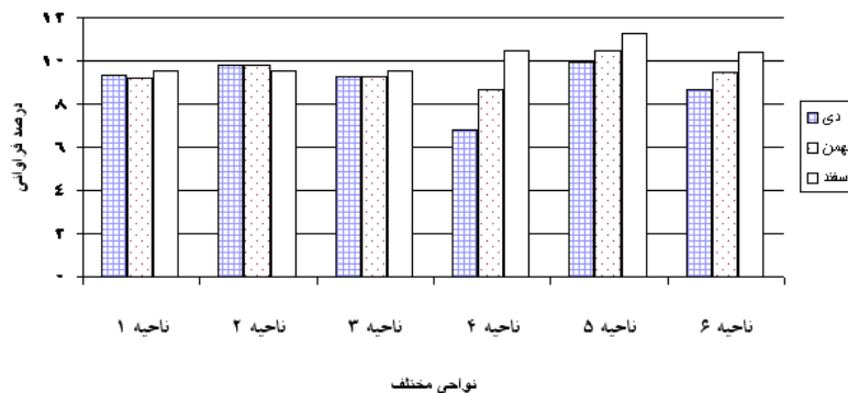
شکل ۱۶) توزیع فراوانی رویدادهای بارشی در نواحی مختلف در ماه‌های فصل زمستان
