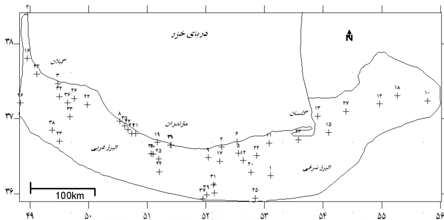
شکل (۱) موقعیت جغرافیایی ۴۶ ایستگاه منتخب همدیده، اقلیم شناسی و باران سنجی در سواحل جنوبی خزر
