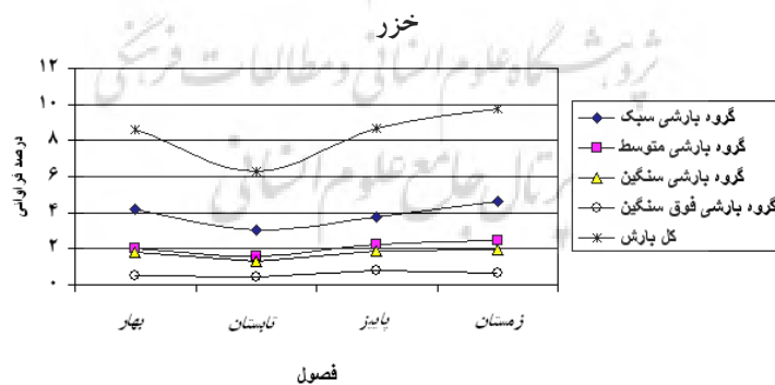
شکل ۱۸) رژیم فصلی میانگین فراوانی رویدادها در گروه‌های مختلف بارشی در سواحل جنوبی
