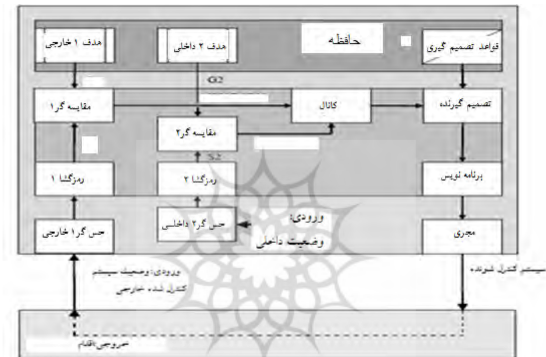
شکل شماره ۵: ساختار یک سطحی سیستم انطباق‌گر
