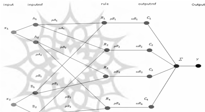
شکل ۲: مدل نهایی برنامه‌ریزی استراتژیک فناوری مبتنی بر نورو - فازی برای هر ماتریس
