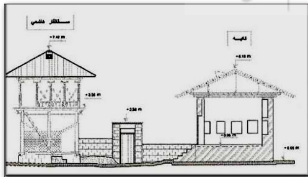
تصویر ۶. مقطع از تکیه و سقانفار در یک مجموعه. مأخذ: پیرزاد، ۱۳۸۷. Fig6. Section of “Tekyeh and Saghanefar” in the collection. Source: Pirzad, 2009.
