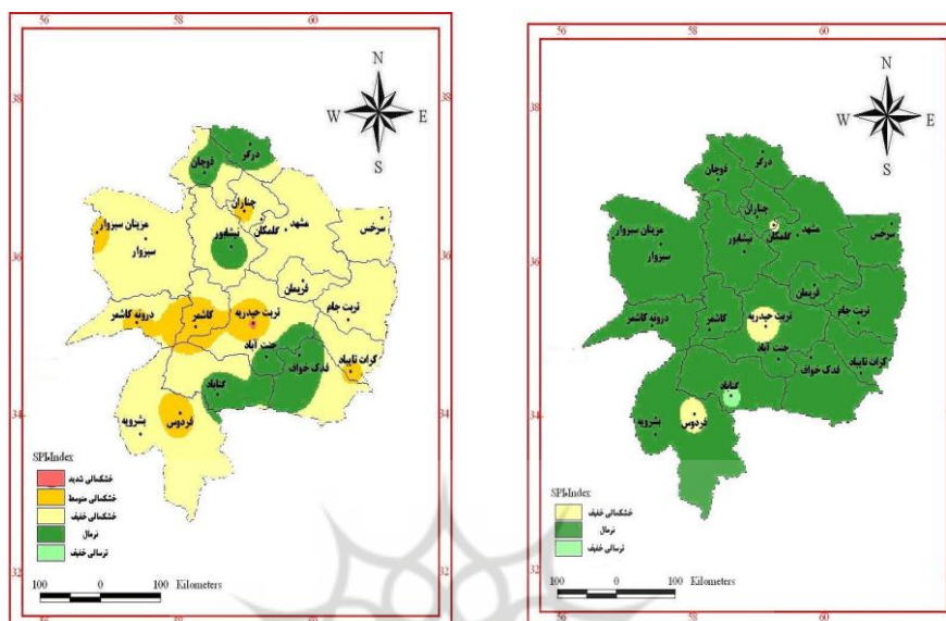
شکل ۷. پهنه بندی شاخص SPI در سال ۱۳۸۵
