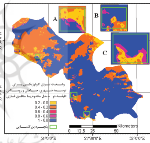
شکل ۱۸. نقشه تناسب برای توسعه شهری طبقه ۲ (منطق فازی)
