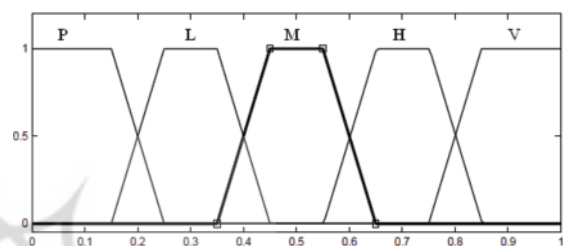
شکل ۸. تابع عضویت فازی تناسب فاکتورهای برای کاربری‌ها
