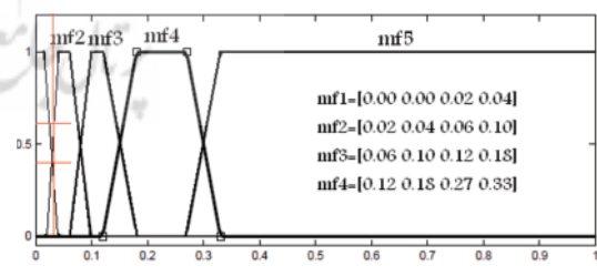
شکل ۹. میزان تعلق شیب ۳/۲ درصد به توابع
