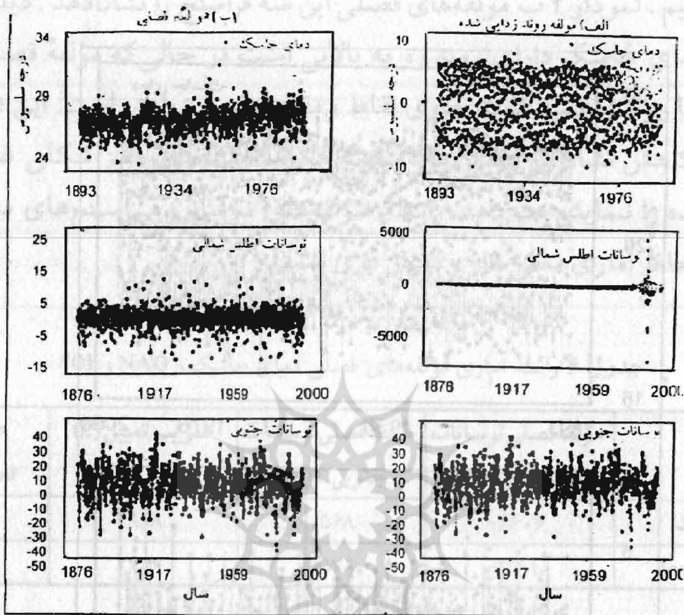
نمودار ۴ مقادیر روندزدایی شده (الف) و مؤلفه‌های نوسانی (ب) دمای جاسک SOI, NAO
