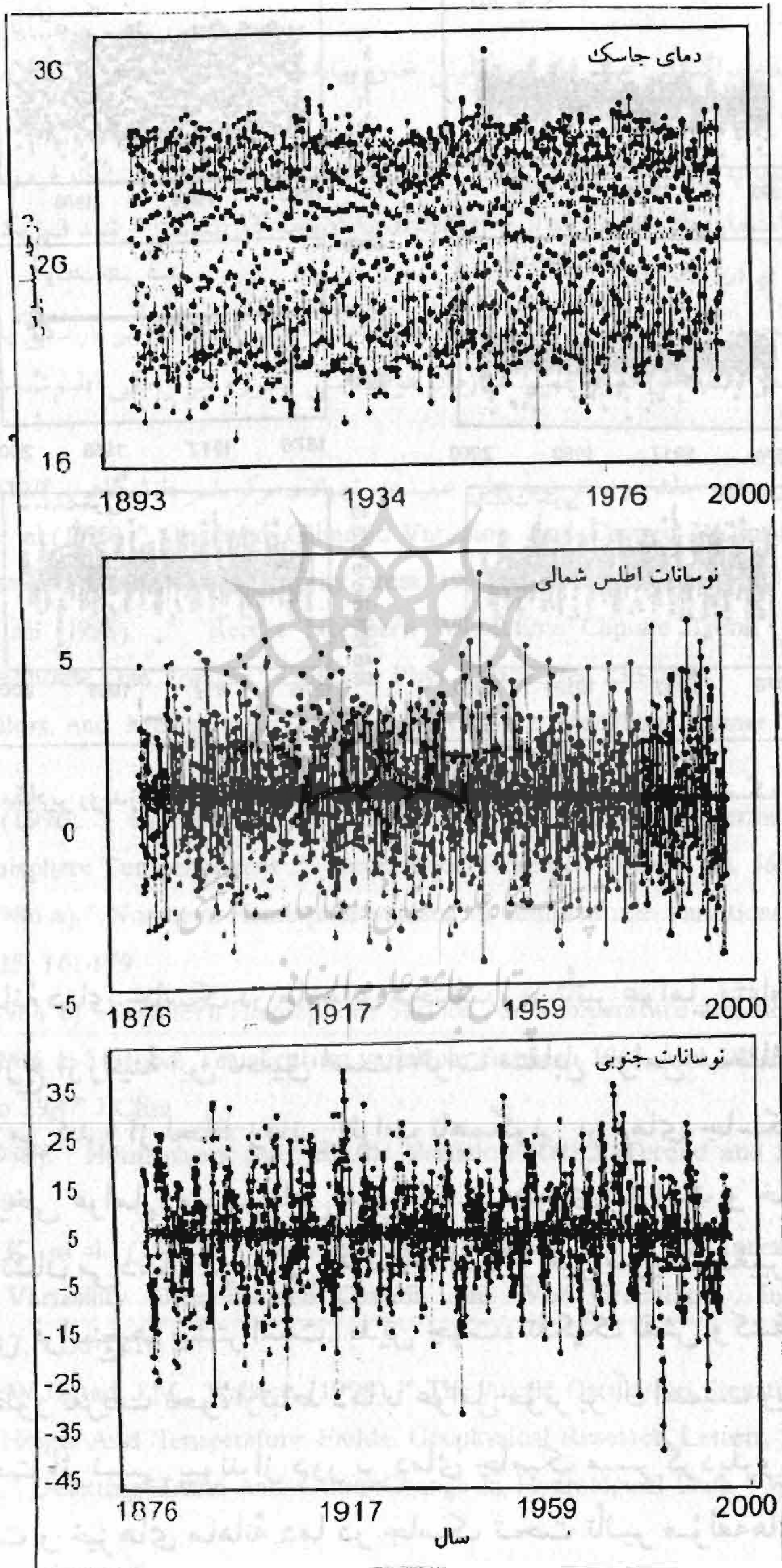
نمودار ۳ میانگین ماهانه و روند بلندمدت دمای جاسک، SOI, NAO
