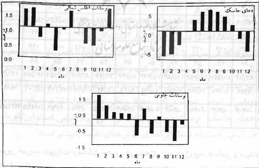
نمودار ۲ شاخص‌های نوسانی دمای جاسک، NAO، SOI
