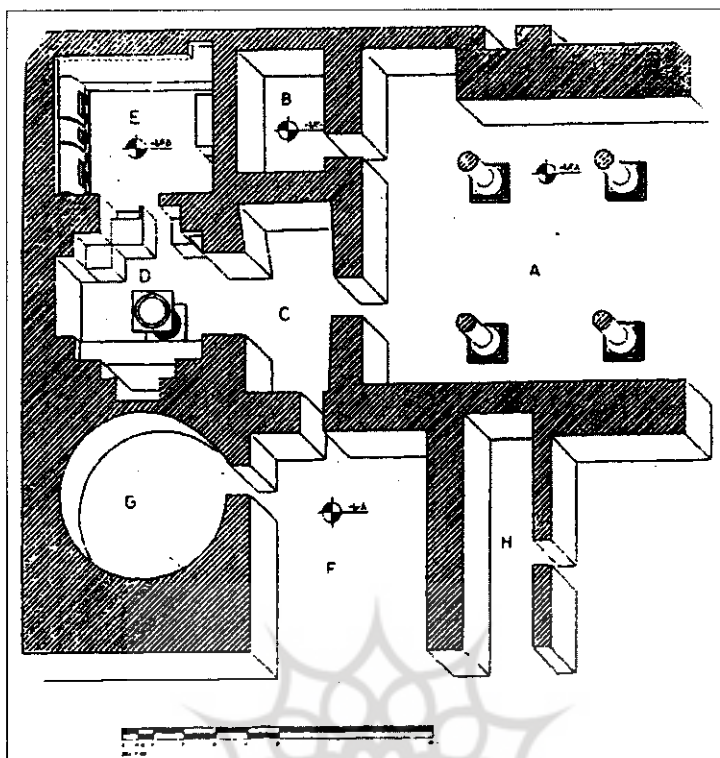
تصویر ۵- طرح ایزومتریک از سازه بندیان با آتشدان، بنگرید به: M. RAH BAR, DE COUVERTE DE PANNEAUX DE (۱۳. P., ۱۹۹۹, MAI, ۲۱۳, STUES SASSANIDES A DARGAZ DOSSIERS D'ARCHEOLOGIE N
