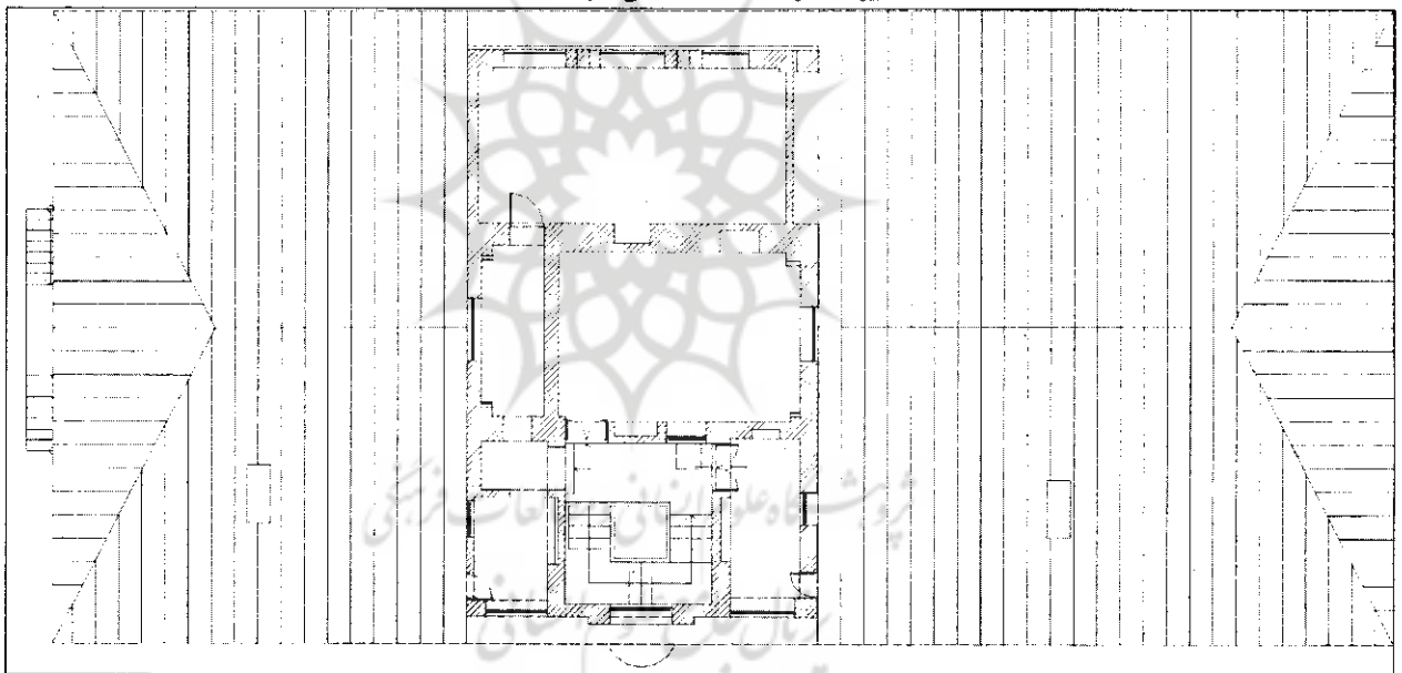
۲. دبیرستان کزازی - ساختمان اصلی - (طبقه اول)
