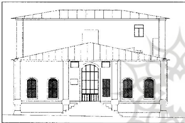
۶. دبیرستان کزازی - ساختمان اصلی - (نمای شرقی)
