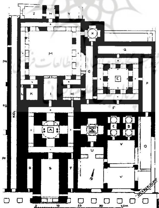
تصویر ۶- پلانی از آتشکده آذرگشنسب، تخت سلیمان، بنگرید به: R. NAUMANN, DIE RUINEN VON TACHT) (۲۴. ABB., ۱۹۷۷, SULEIMAN UND ZENDAN-E SULEIMAN, BERLIN
