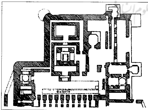
تصویر ۱: پلان آتشکده کوه خواجه، بنگرید به (M.MOUS WILKHEH-E KHADJEH), UN COMPLEXE RELIGIEUX DE L'EST IRANIEN, DOSSIERS D'ARCHÉOLOGIE N 243, MAI 1993, P.83)
