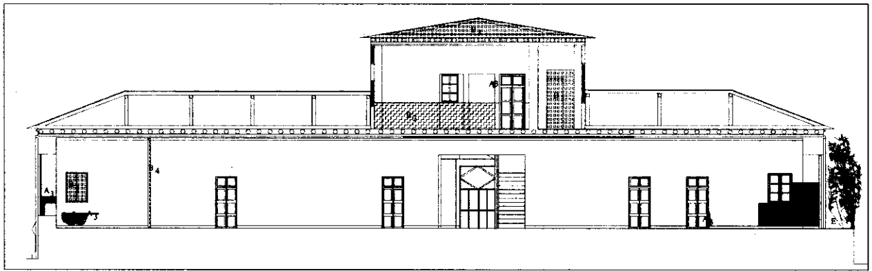
۴. دبیرستان کزازی - ساختمان اصلی - (برش طولی)
