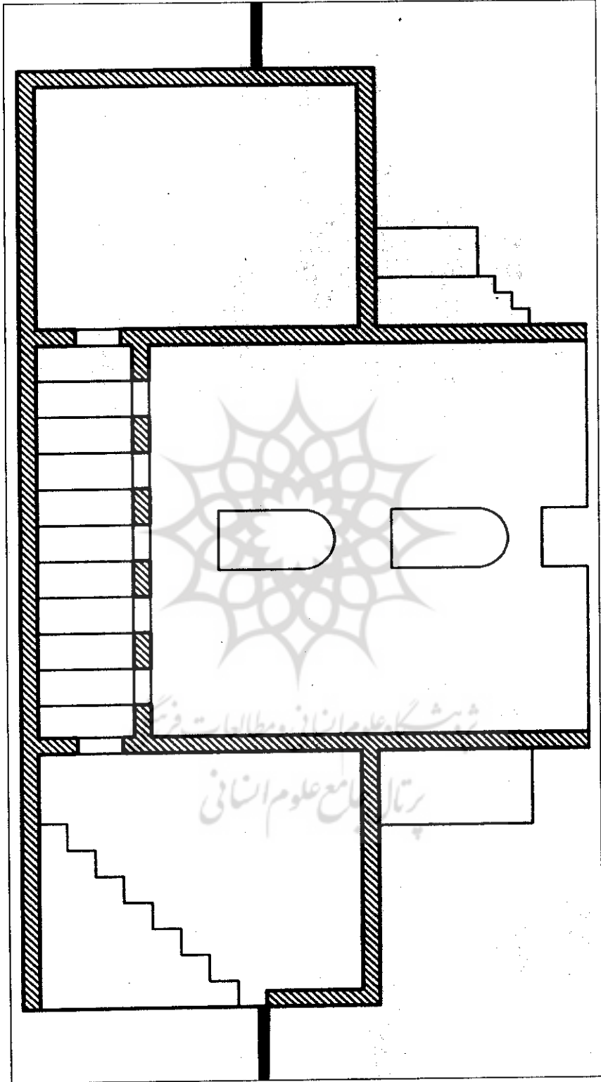
شکل ۱۰: برش نمونه‌ای از کوره‌های آجرپزی چاه‌نیم منطقه دزفول - خوزستان
