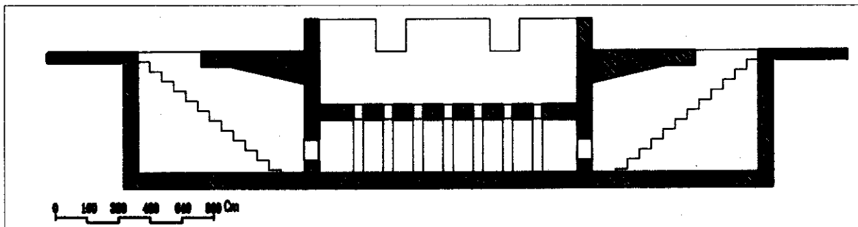
شکل ۷: برش نمونه‌یی از کوره‌های از نوع چاله‌ای منطقه شوش - خوزستان
