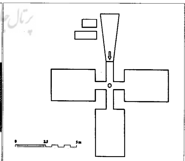
شکل ۳: پلان و مقطع نمونه‌یی از کوره‌های منطقه گز برخوار - اصفهان
