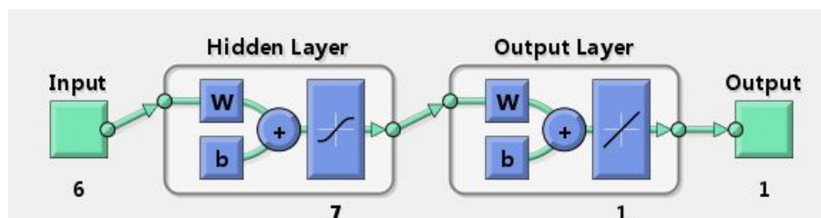
شکل 1- طراحی شبکه عصبی مصنوعی با متغیر خروجی ضریب جینی شهری
