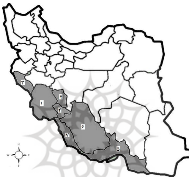
شکل ۱- استانهای واقع در جنوب و جنوب غربی ایران (۱- خوزستان، ۲- چهار محال بختیاری، ۳- ایلام، ۴- کهگیلویه و بویراحمد، ۵- هرمزگان، ۶- فارس، ۷- بوشهر)
