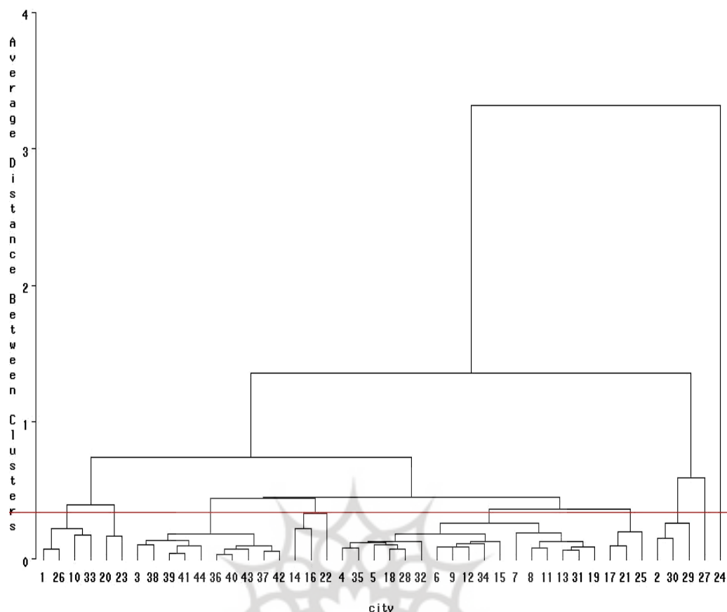
شکل ۳- دندروگرام حاصل از انجام تجزیه خوشه ای به روش Average برای ۴۴ ایستگاه سینوپتیک واقع شده در جنوب و جنوب غرب ایران (برش دندروگرام در محلی است که ۹ پهنه اقلیمی مشاهده گردد).
