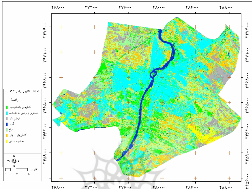
شکل ۳. طبقه‌بندی نظارت‌شده تصویر سال ۱۹۹۱ با استفاده از الگوریتم بیشترین همبندی
