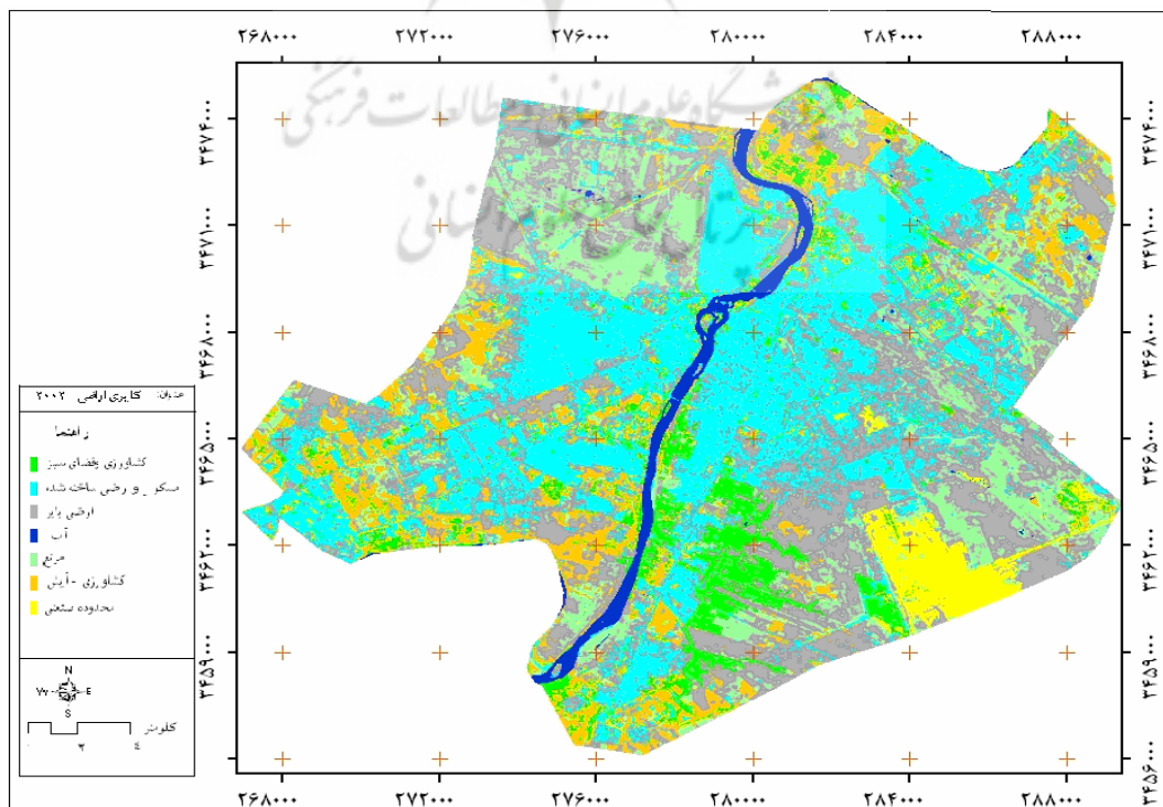
شکل ۴. طبقه‌بندی نظارت‌شده تصویر سال ۲۰۰۲، با استفاده از الگوریتم بیشترین همبندی
