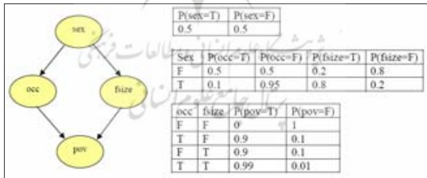
شکل ۲: ساختار شبکه بیزی با ۴ گره و جداول احتمال مربوط به آن
