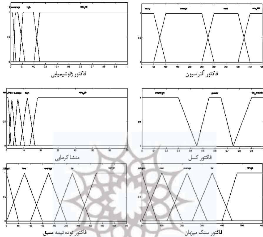
شکل ۳ توابع عضویت فازی فاکتورهای ورودی
