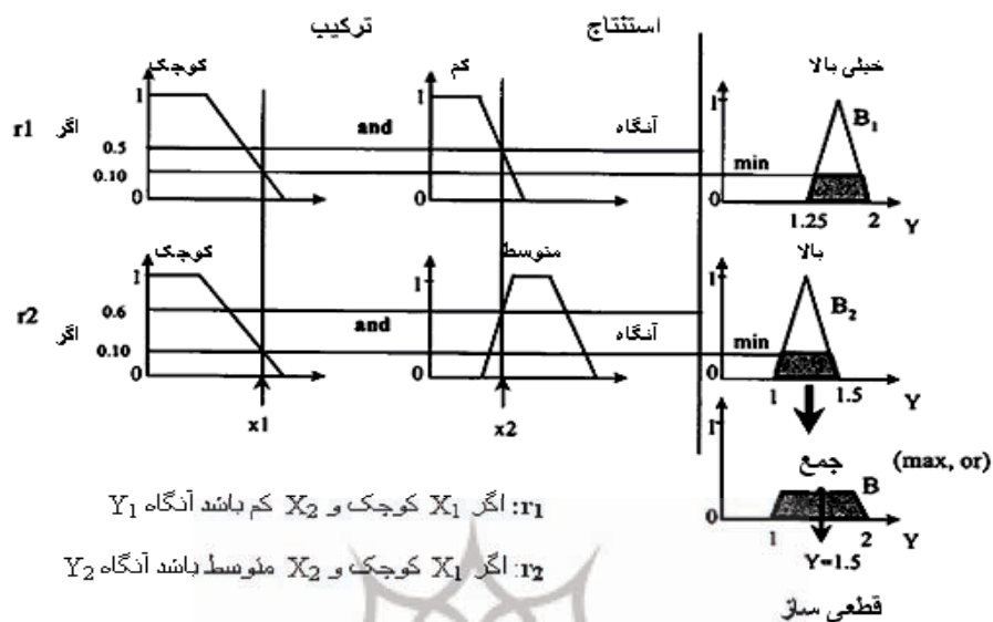
شکل ۵ نمایی شماتیک از مکانیزم استنتاج فازی مدل ممدانی با دو قاعده
