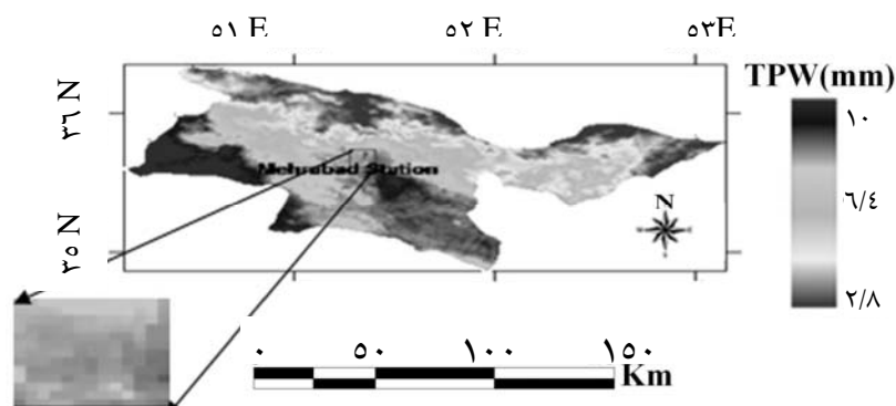
شکل ۸ آب قابل بارش کلی حاصل از باند ۱۹ به ۲ در گذر ۲۶ می ۲۰۰۳
