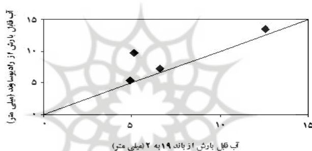
شکل ۹ مقایسه بین آب قابل بارش به دست آمده از نسبت باند ۱۹ به ۲ و آب قابل بارش محاسبه شده از داده‌های رادیوساوند
