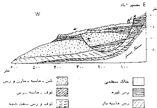
شکل ۲. مقطع شوماتیک لغزش نصیرآباد
