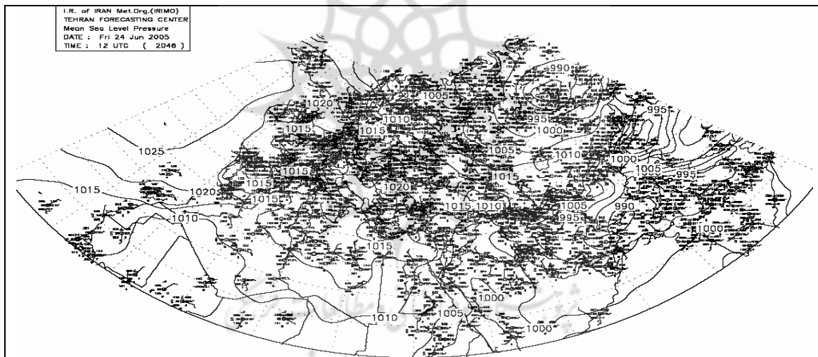
شکل ۶ شرایط سینوپتیکی تراز متوسط دریا در روز ۲۴ ژوئن ۲۰۰۵
