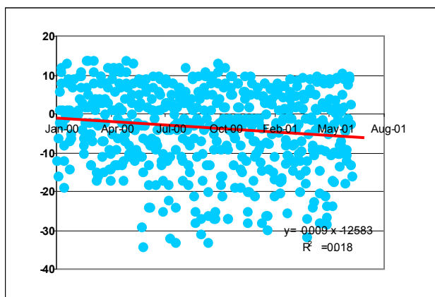
شکل ۳ روند تغییرات دمای نقطه شبم ماهانه ایستگاه تهران (۱۹۹۵-۱۹۹۸)
