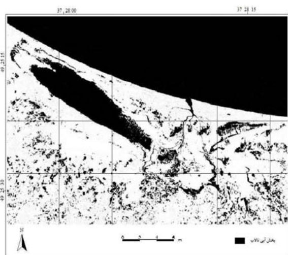
شکل شماره (۱): تبدیل تصویر ماهواره‌ای سال ۱۹۹۱ به دو طبقه آب و خشکی
