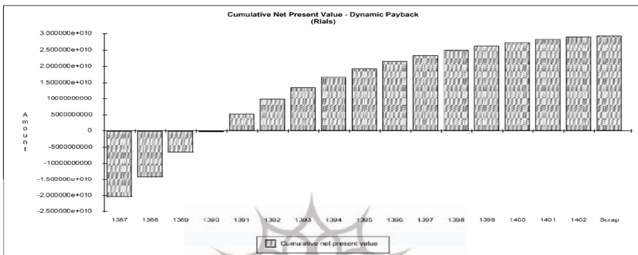
شکل شماره (۶): نمودار دوره بازگشت سرمایه به صورت دینامیک در Plant B با استفاده از نرم افزار اقتصادی COMFAR
