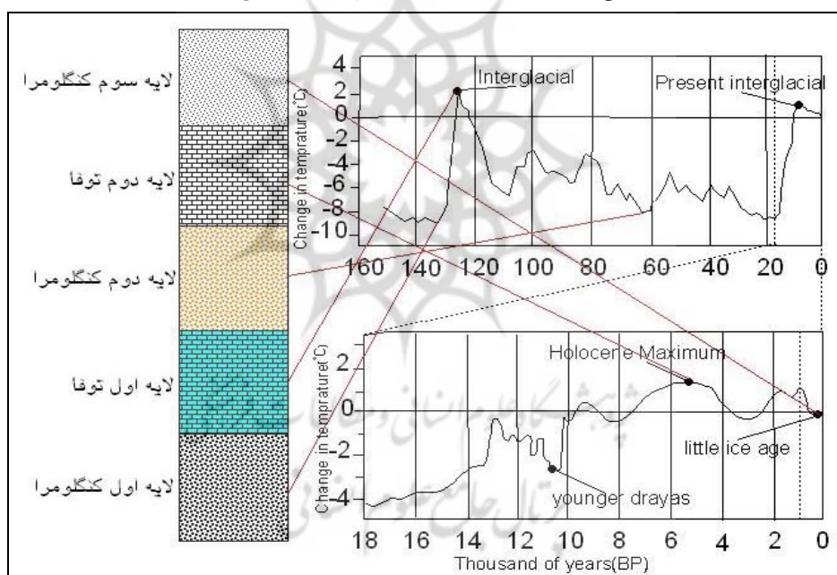
شکل ۱۱- تطبیق لایه‌های تشکیل دهنده مخروط افکنه با تقویم تغییرات اقلیمی (Siegert, 2001: 2).
