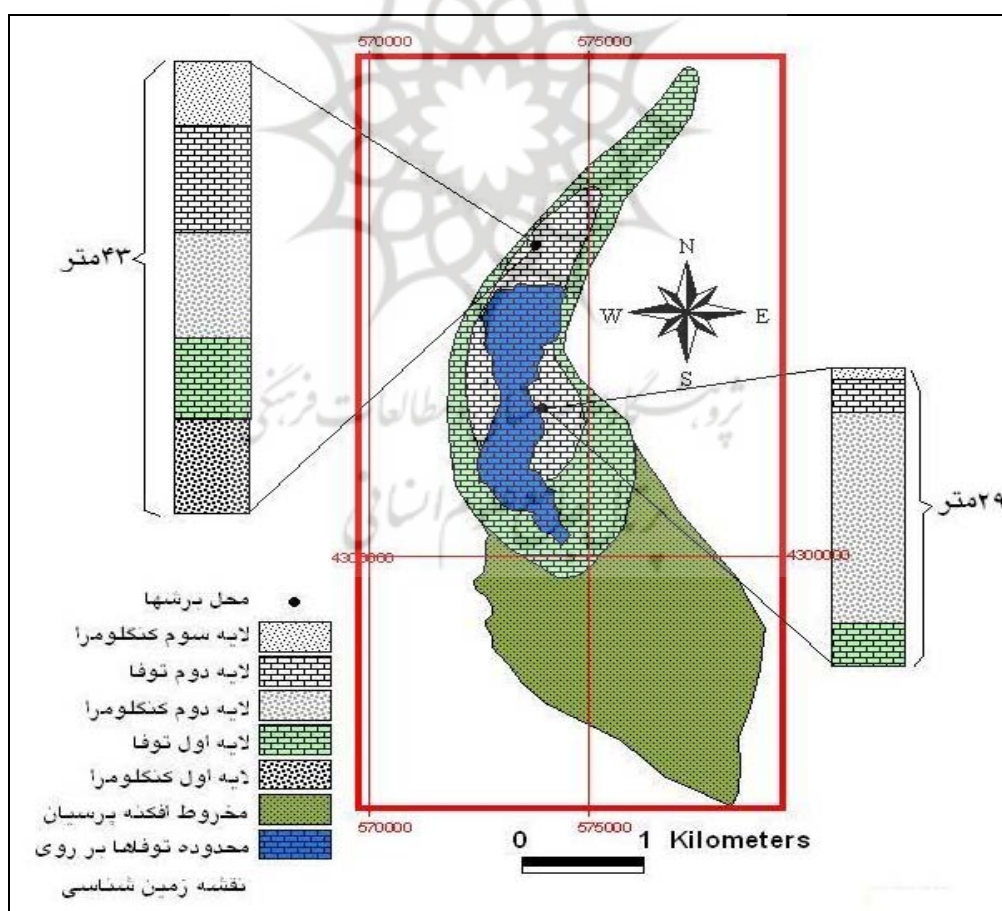
شکل ۳- محدوده نهشته‌های توفایی در پایین دست مخروط افکنه پرسیان، لازم به یاد آوری است که تعیین محدوده لایه اول و دوم توفاف بر اساس ردیابی این نهشته‌ها بر روی زمین و با استفاده از GPS صورت گرفته است.
