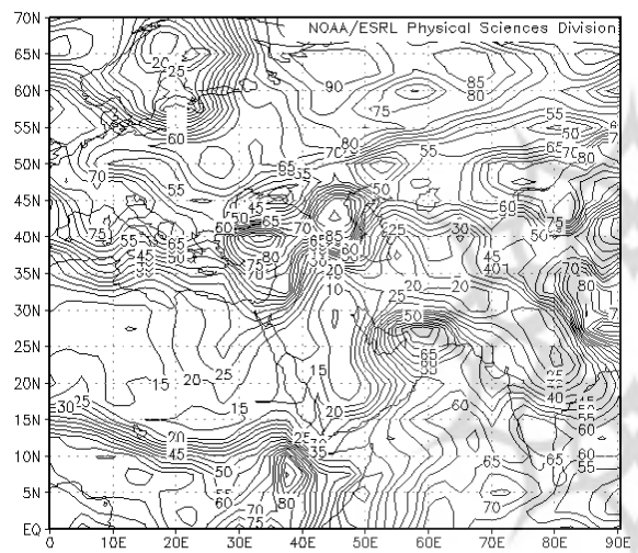
و(روز هشتم سطح ۸۵۰ هکتوپاسکال
