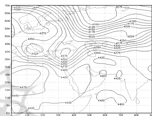
ن) روز هشتم. سطح ۶۰۰ هکتوپاسکال
