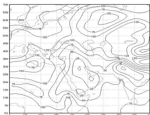
ل) روز هشتم. سطح ۱۰۰۰ هکتوپاسکال
