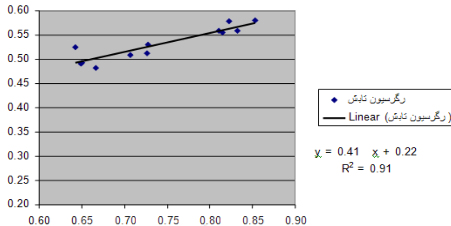
نمودار شماره (3) مدل نهایی رگرسیون بین \frac{\bar{H}}{\bar{H}_0} و \frac{\bar{S}}{\bar{S}_0}
