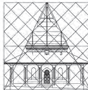
تصویر ۳۰ - شبکه خطوط ۴۵ درجه ای که اساس طرح هندسی گنبد را تشکیل می دهند، در صورتی که توسعه داده شود و تمام مربع زمینه را فراگیرد، نمای ایوان ورودی را هم به شش قسمت مساوی تقسیم می کند و موقعیت ستونها را در آن تعریف می کند و این امر می تواند تأییدی باشد برای این فرضیه که طراح، در طرح بنا از این شبکه هندسی استفاده کرده است.
