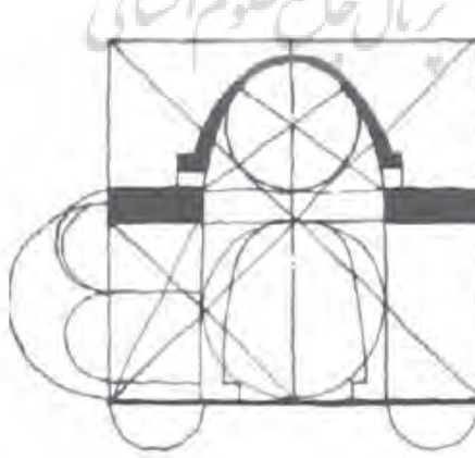
تصویر ۱۶- هندسه در چهارطاق ورجاوند. مأخذ: (اردلان, ۱۳۷۹, ۲۳)
