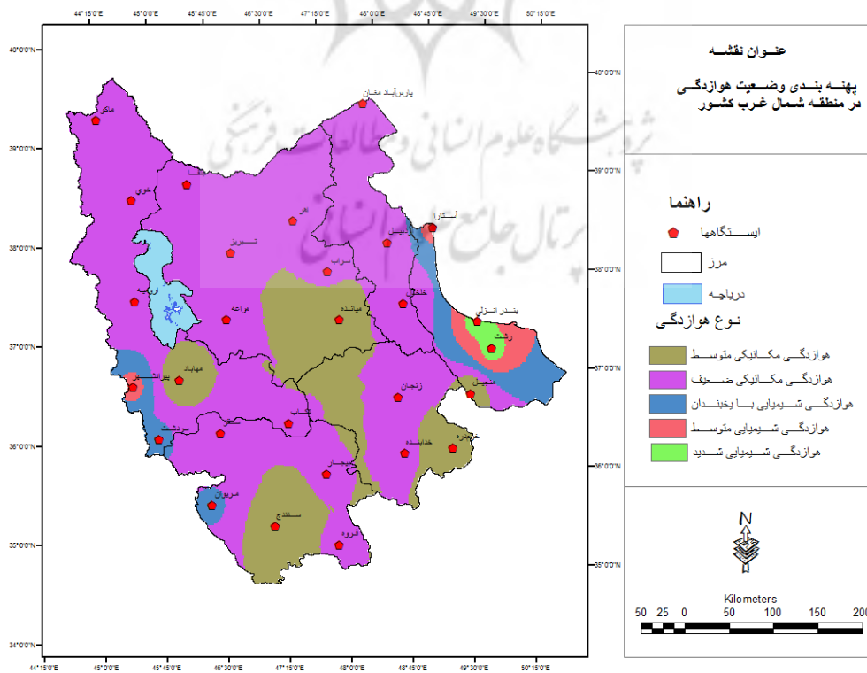
شکل ۷. طبقه‌بندی نوع و شدت هوزدگی، براساس مدل پلتیر در شمال غرب کشور (دوره آماری ۲۰۰۵-۱۹۷۶)
