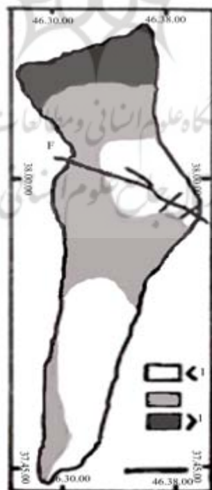
شکل ۱۲. سطوح هم‌ارزش شاخص V_f در حوضه سعیدآبادچای
