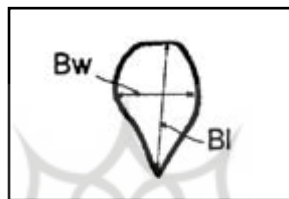
شکل ۷. رابطه نسبت شکل حوضه زهکشی
