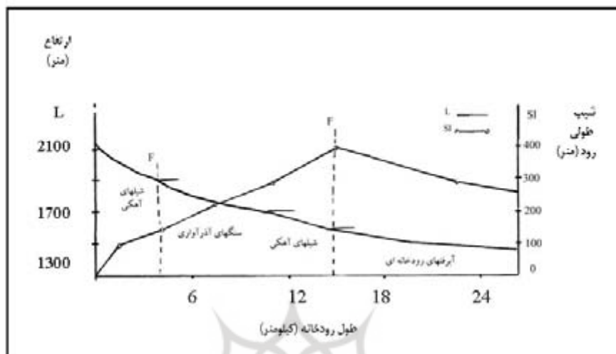
شکل ۴. نیمرخ طولی و نمودار تغییرات شیب رودخانه در زیرحوضه کندولچای L: نیمرخ طولی رودخانه SL: مقادیر شاخص F: گسل
