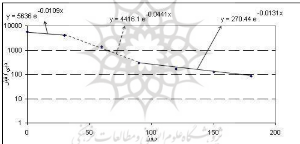
شکل ۳-۲. منحنی تاریخچه سراب برناج
