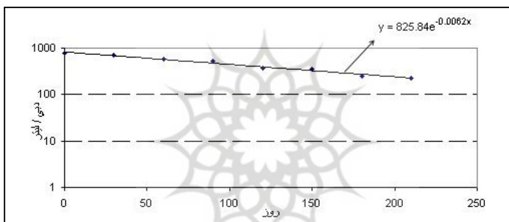
شکل ۳-۵. منحنی تاريسمان سراب نیلوفر
