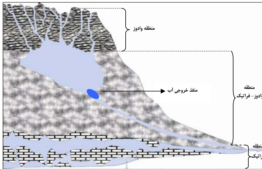
شکل ۴. طرح شماتیکی از بستر تغذیه چشمه‌های کارستی در توده پرآو - بیستون
