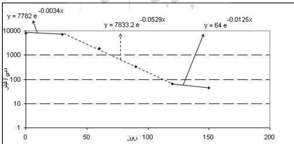
شکل ۳-۳. منحنی تاریخچه سراب طاق بستان
