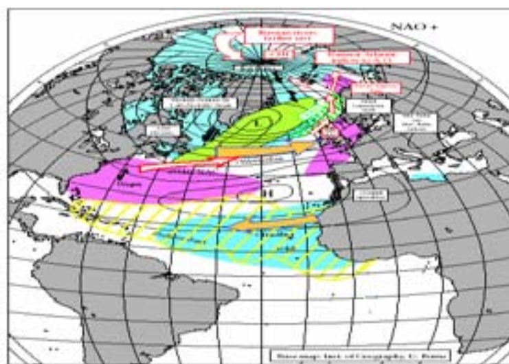
شکل ۲ جهت جریان و نحوه استقرار پرفشار آزرز و کم فشار ایسلند طی فاز مثبت NAO (از موسسه جغرافیایی برنی، اینترنت)
