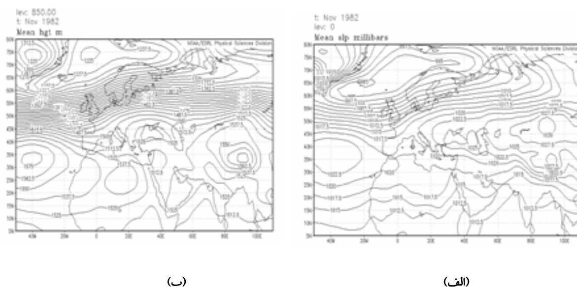
شکل ۷ نقشه سطح متوسط دریا و تراز ۸۵۰ هکتوپاسکال، طی فاز مثبت (نوامبر ۱۹۸۲)
