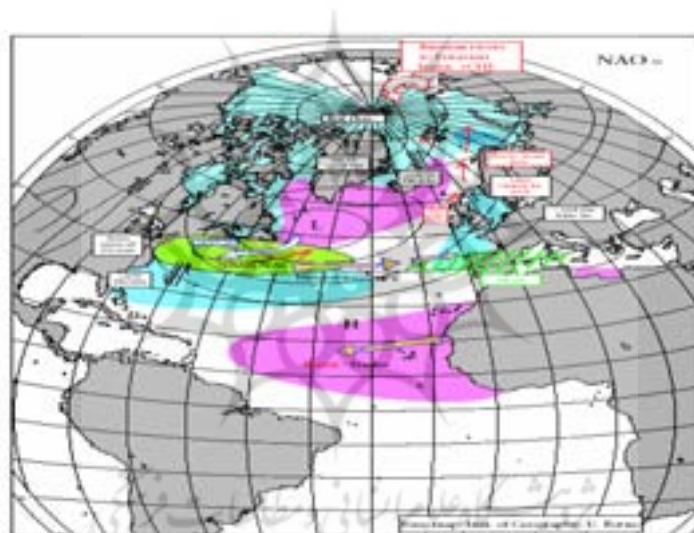
شکل ۳ جهت جریان و نحوه استقرار پرفشار آزرز و کم فشار ایسلند طی فاز منفی NAO (از موسسه جغرافیایی برنی، اینترنت)
