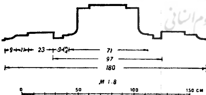
پلان محراب اسکادر
