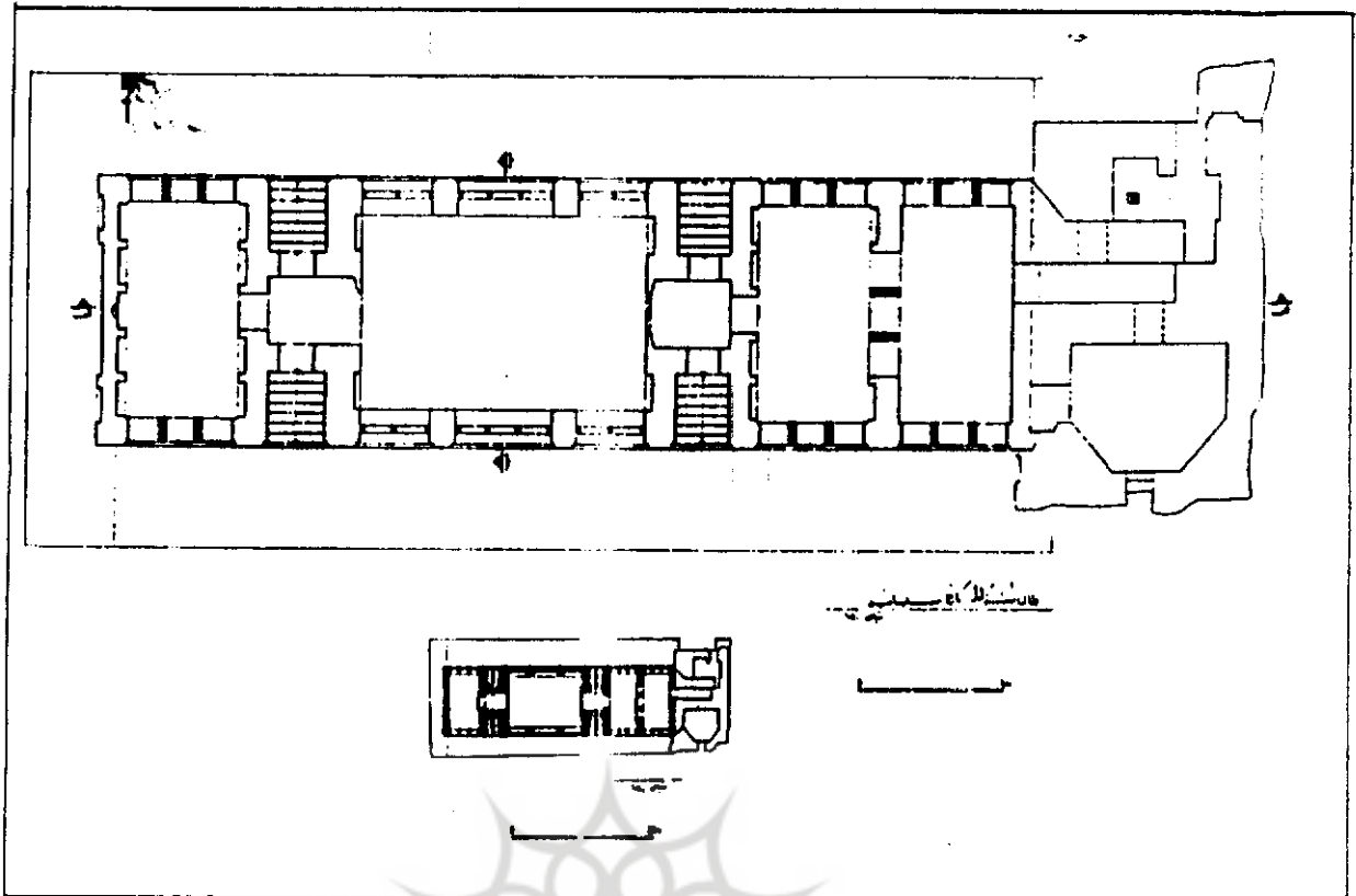
نقشه ۴ - آثار بازمانده از برج مجاور کاخ در طبقه اول
