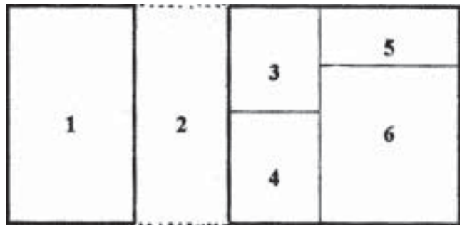
پلان طبقه همکف نخستین مسجد در شهر برادفورد، انگلستان ۱. زیرزمین ۲. راه سرپوشیده به پشت مسجد ۳. سرویس بهداشتی ۴. آشپزخانه ۵. کفش کن ۶. وضوخانه
