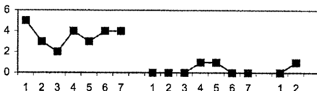
نمودار ۶ - فراوانی میزان بی اجازه صحبت کردن آزمودنی سوم در کلاس ریاضی در سه مرحله خط پایه، مداخله و نگهداری
