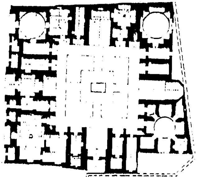
پلان مدرسه دو در (طبقه همکف)
