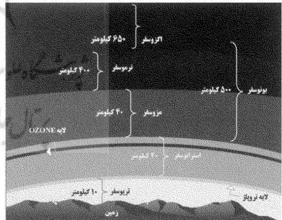
نگاره ۱: لایه‌های جو زمین
