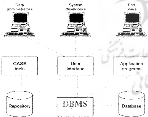
نگاره ۱: تشکیلات و بخش‌های مختلف موجود در یک سامانه مبتنی بر پایگاه داده
