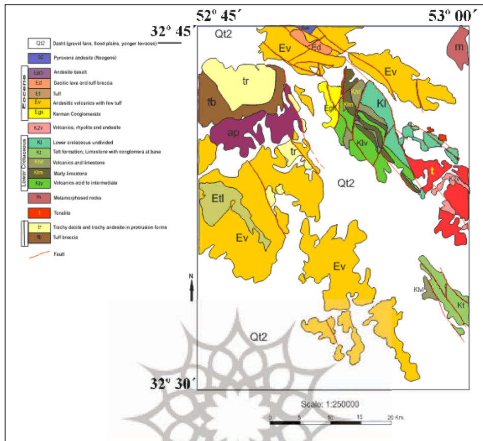
شکل ۲. نقشه زمین‌شناسی منطقه مورد مطالعه برگرفته از نقشه‌ی نائین با مقیاس ۱:۲۵۰۰۰۰ با اندکی تغییرات.
