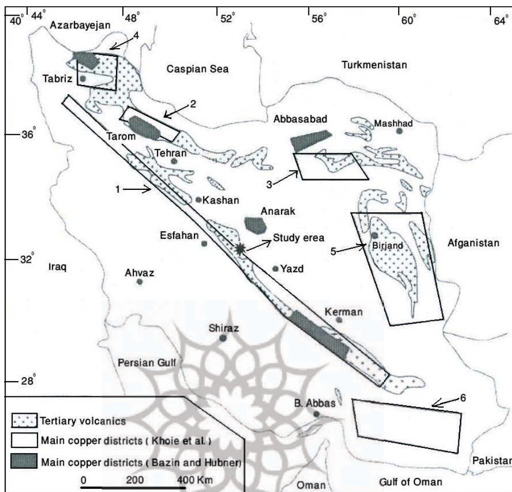
شکل ۱. زونهای اصلی کانسارسازی مس در ایران. کانسارهای مس ایران در شش منطقه یا زون جغرافیایی رخ داده است که عبارتند از: ۱- زون آتشفشانی ارومیه- دختر ۲- زون البرز باختری ۳- زون کویر- سبزواری ۴- زون سبلان ۵- زون لوت ۶- زون مکران.
