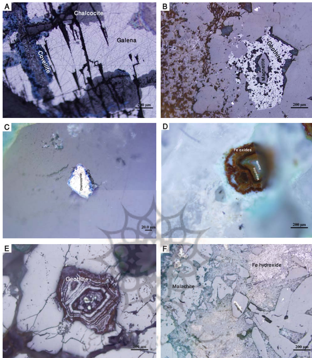
شکل ۳. تصاویر میکروسکوپی از مقاطع صیقلی. A: پارازنز گالن، کالکوسیت و کوولیت و جهت‌یافتگی و کشیدگی رخی‌های گالن در اثر تنش‌های تکتونیکی B: تبدیل مگنتیت به گوتیت C: تبدیل کالکوپیریت به کوولیت از حاشیه D: افتادگی یک سمت کانه‌ها در مقطع نسبت به طرف مقابل در اثر تنش‌های تکتونیکی E: تبدیل هماتیت به گوتیت F: تجزیه کالکوپیریت و تشکیل مالاکیت و باقی‌مانده‌هایی از کالکوپیریت به صورت افشان.
